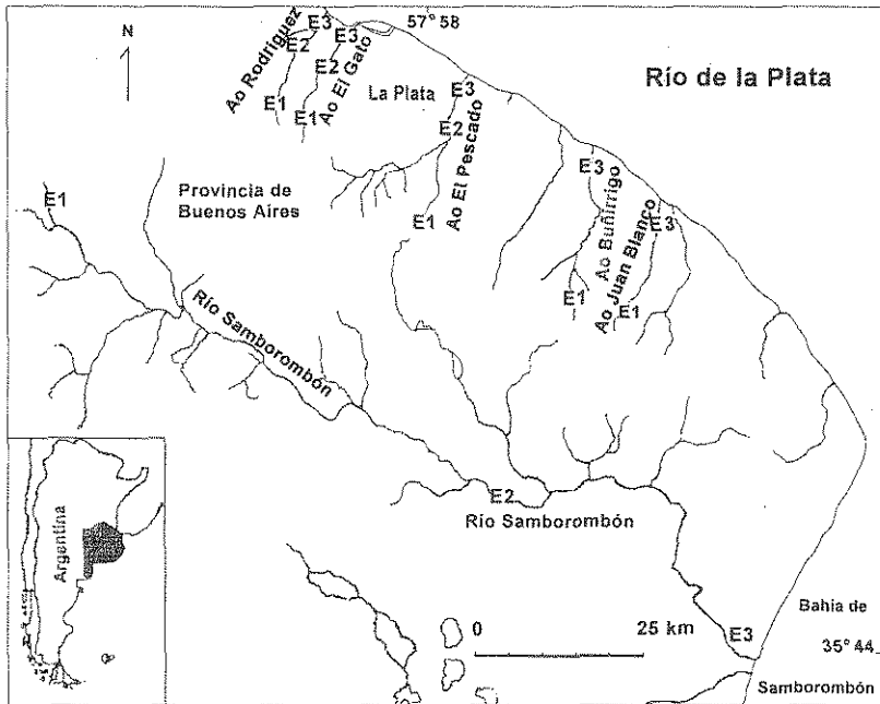
Fig. 1. Ubicación de los arroyos Rodríguez, El Gato, El Pescado, Buñirigo, Juan Blanco y del río Samborombón en el sector NE de la Provincia de Buenos Aires.
