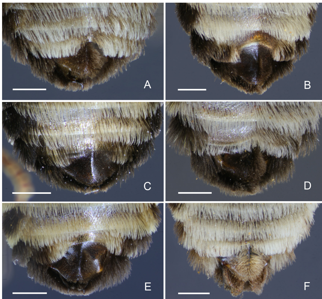
Fig. 7. Apical metasomal sterna of males. A. P. aemulatrix n. sp. B. P. relata . C. P. scalaris . D. P. rubescens n. sp. E. P. plumata . F. P. vulpihirta . Scale bars = 1 mm.
